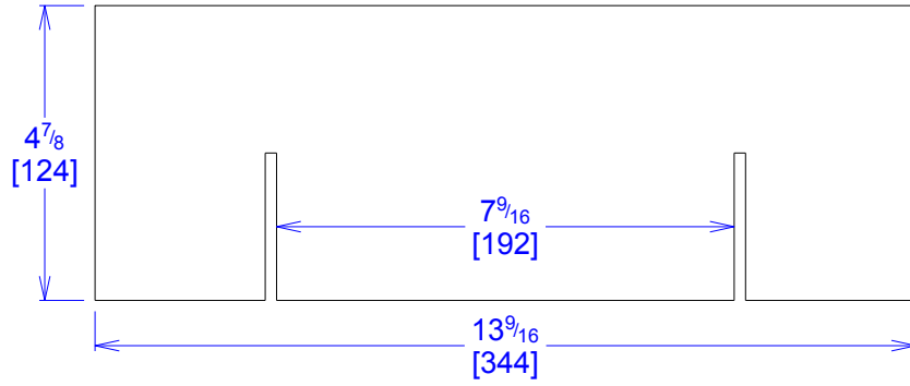
COMPONENTE A 1 PIEZA POR SET
