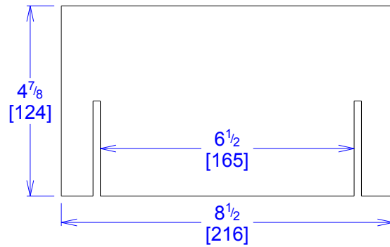
COMPONENTE C 2 PIEZAS POR SET
