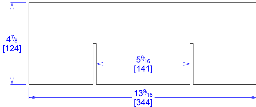
COMPONENTE B 1 PIEZA POR SET
