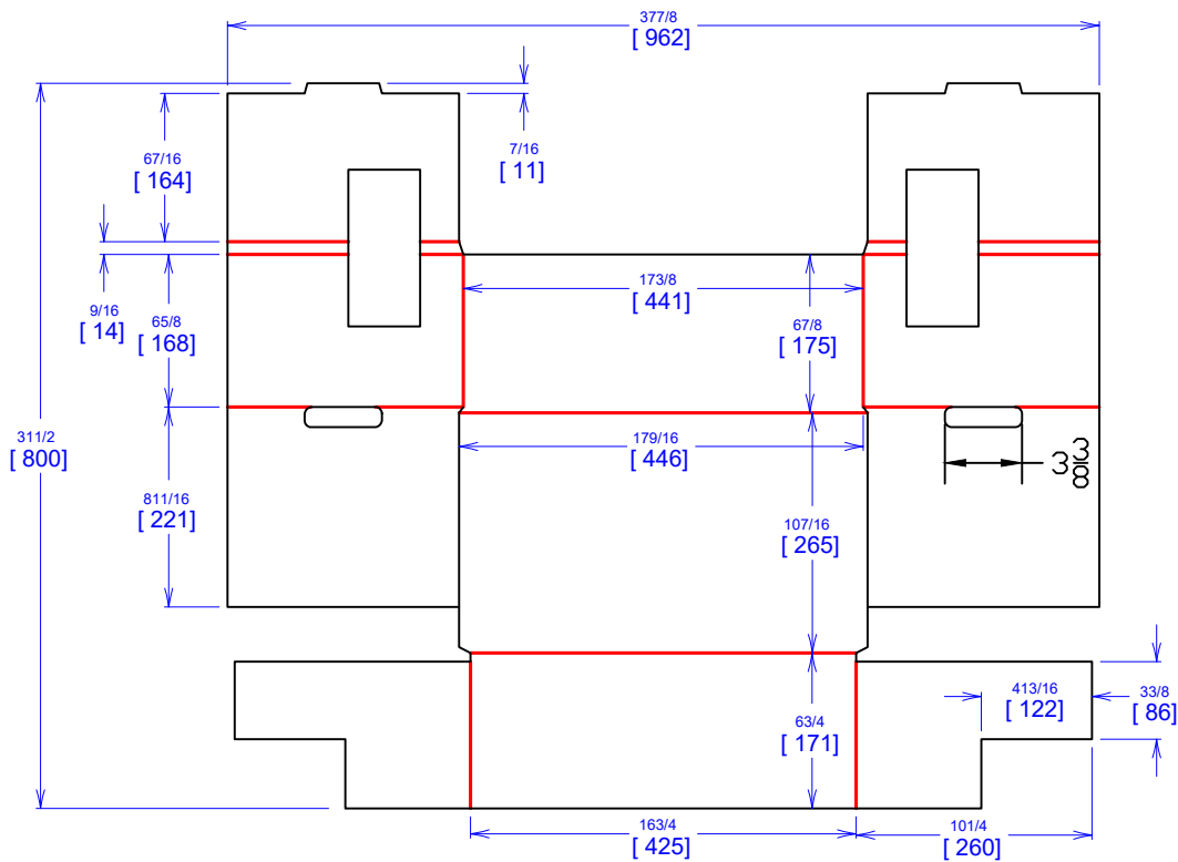
DIMENSIONES EXTERIORES
