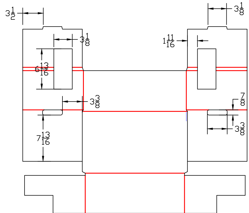
DIMENSIONES INTERIORES
